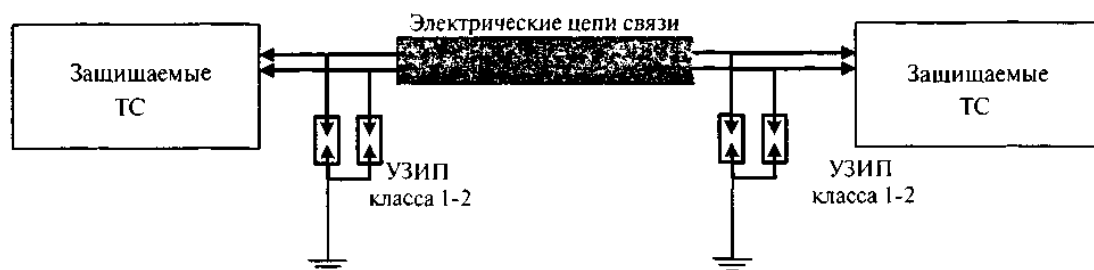
Рисунок 11.3 - Общая схема снижения помех в сигнальных цепях оборудования систем автоматики
