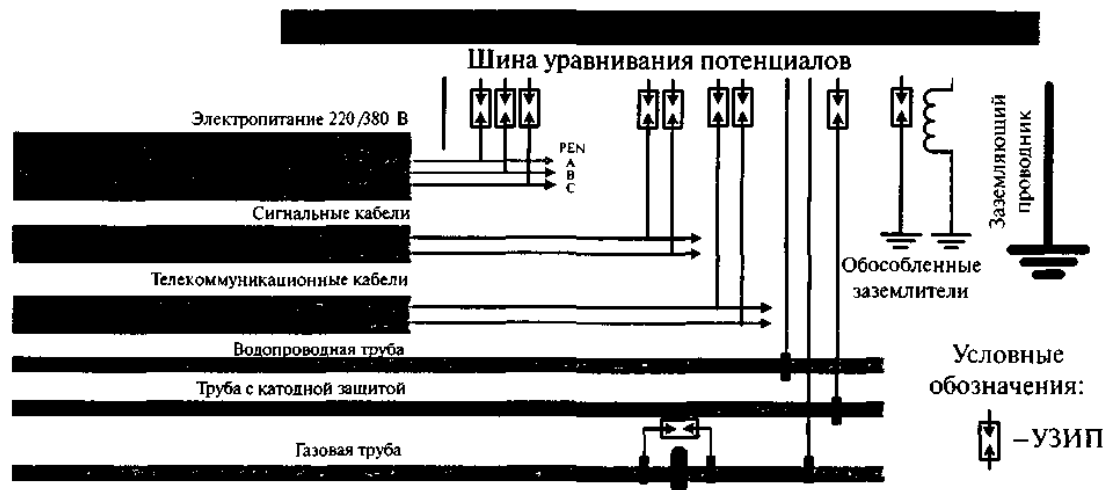
Рисунок 10.1 - Соединение входящих в здание коммуникаций с главной заземляющей шиной
