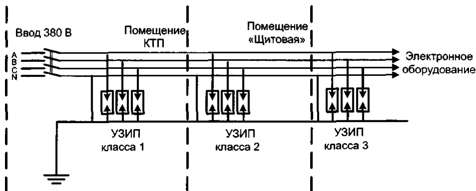
Рисунок Б.1 - Типовая схема установки УЗИП согласно зоновой концепции
