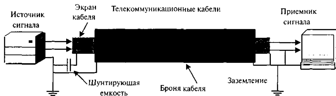
Рисунок 10.4 - Заземление экрана кабеля с использованием шунтирующей емкости
