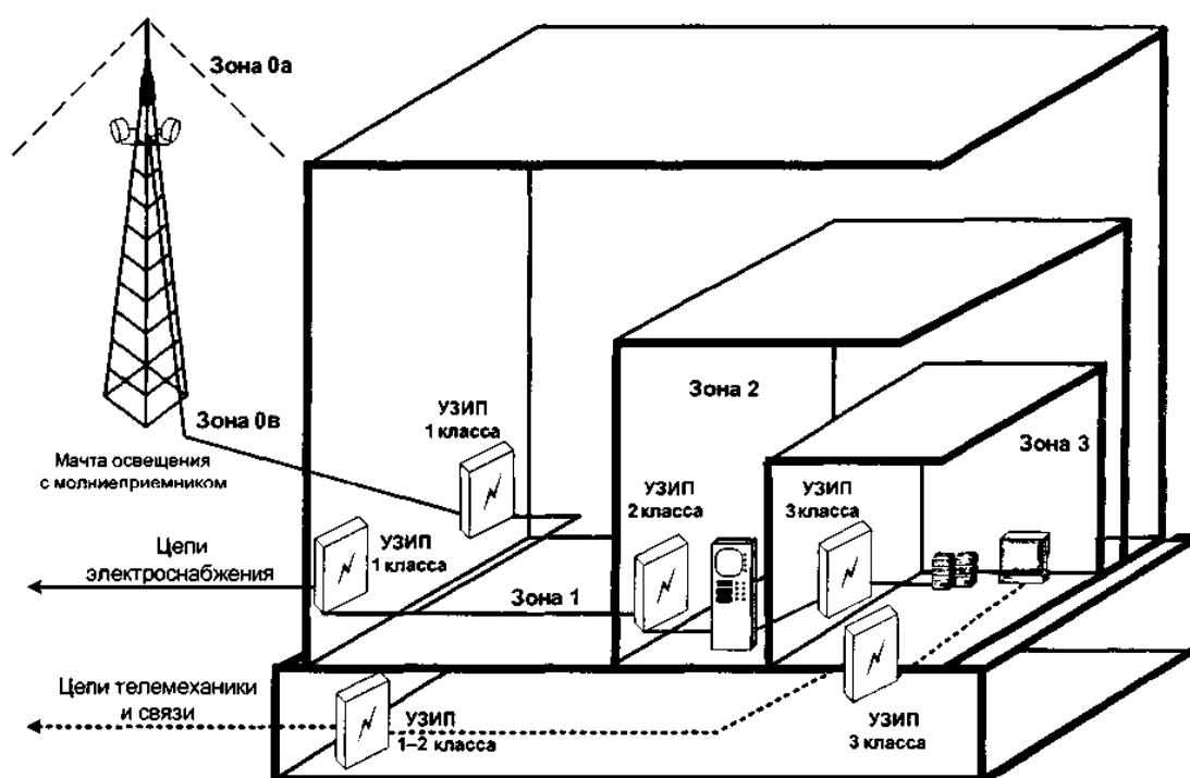
Рисунок 10.2 - Зоны молниезащиты согласно зонной концепции
