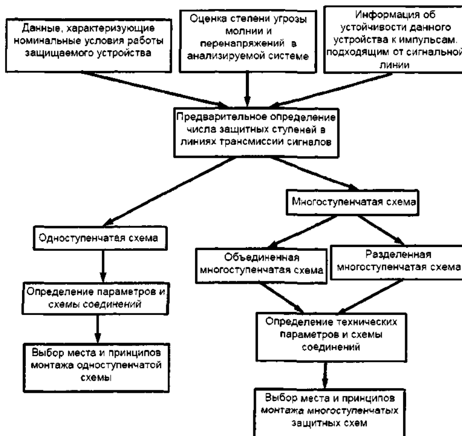
Рисунок 10.3 - Алгоритм действий при выборе УЗИП
